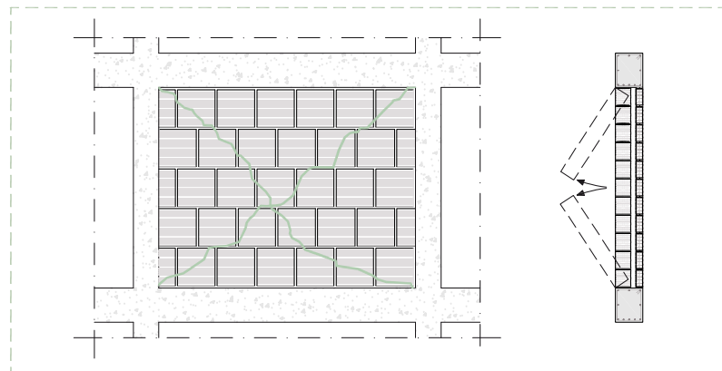
MECANISMO DE COLAPSO 1
