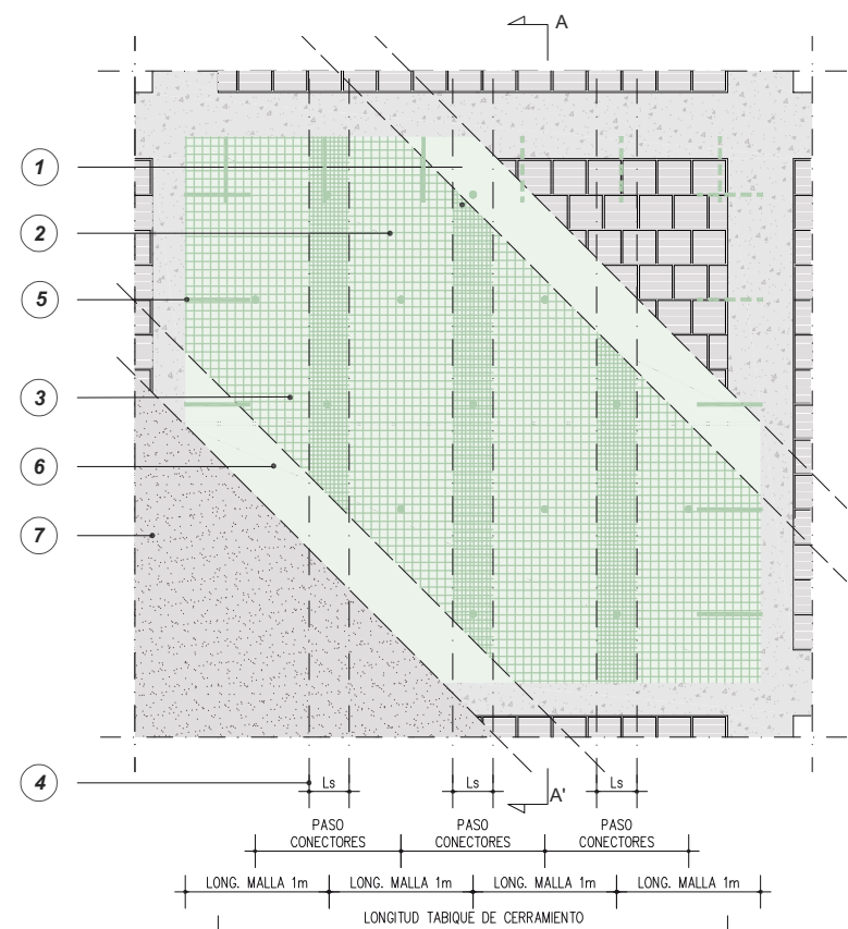
DETALLE SISTEMA DE ENCAMISADO ANTIVUELCO DE CERRAMIENTO CON GEO GRID 120 Y BARRAS STEEL DRYFIX 10
