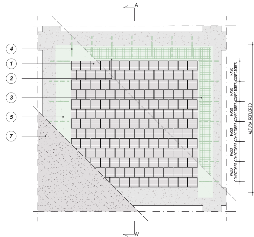
DETALLE REFUERZO DE CERRAMIENTO CON GEO GRID 120 EN COMBINACIÓN CON GEOCALCE F ANTISISMICO Y BARRAS HELICOIDALES DE ACERO INOXIDABLE
