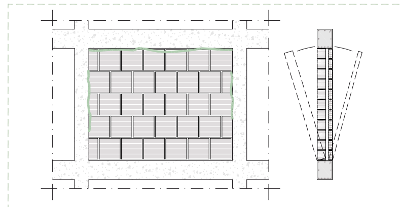
MECANISMO DE COLAPSO 2
