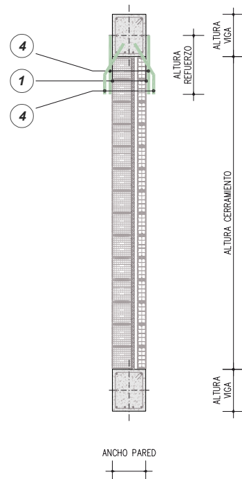
SECCIÓN A - A' REFUERZO DE CERRAMIENTO CON GEO GRID 120 EN COMBINACIÓN CON GEOCALCE F ANTISISMICO Y BARRAS HELICOIDALES DE ACERO INOXIDABLE
