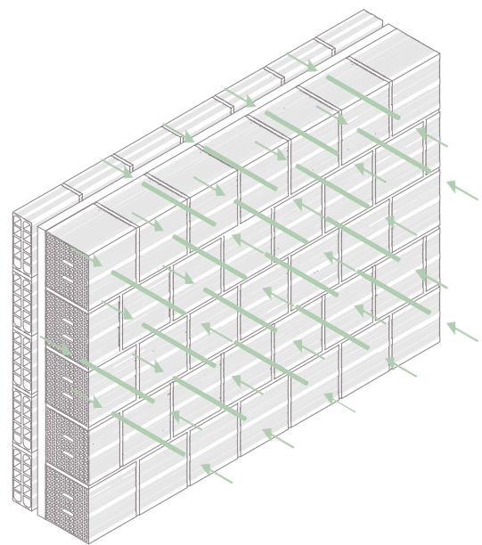
VISTA AXONOMÉTRICA COSIDO EN SECO CON BARRAS HELICOIDALES
