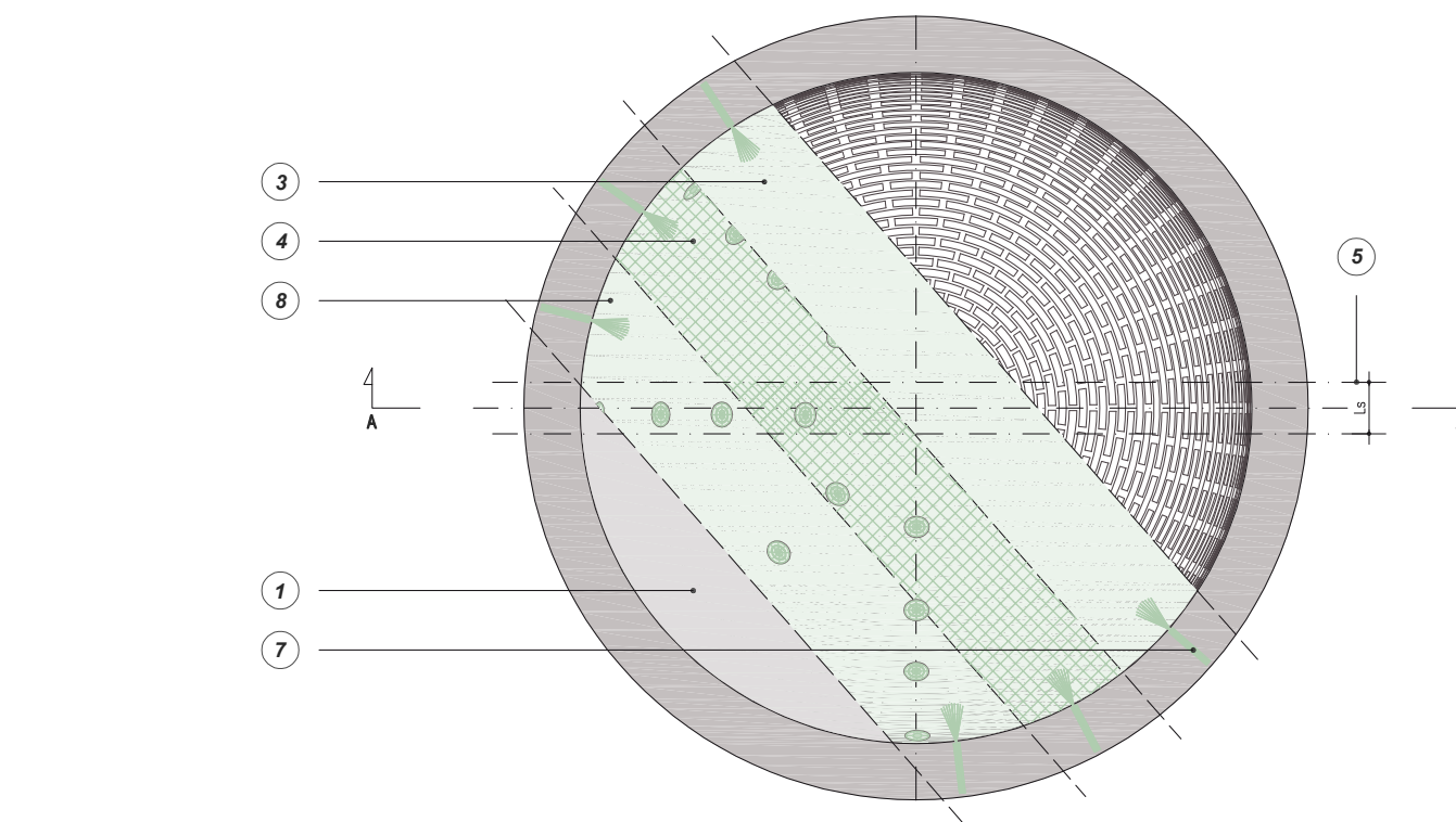
PIANTA B-B' SISTEMI DI RINFORZO ALL'INTRADOSSO CON RETE DIFFUSA GEOSTEEL GRID 200/400 O RINFORZO ARV 100
