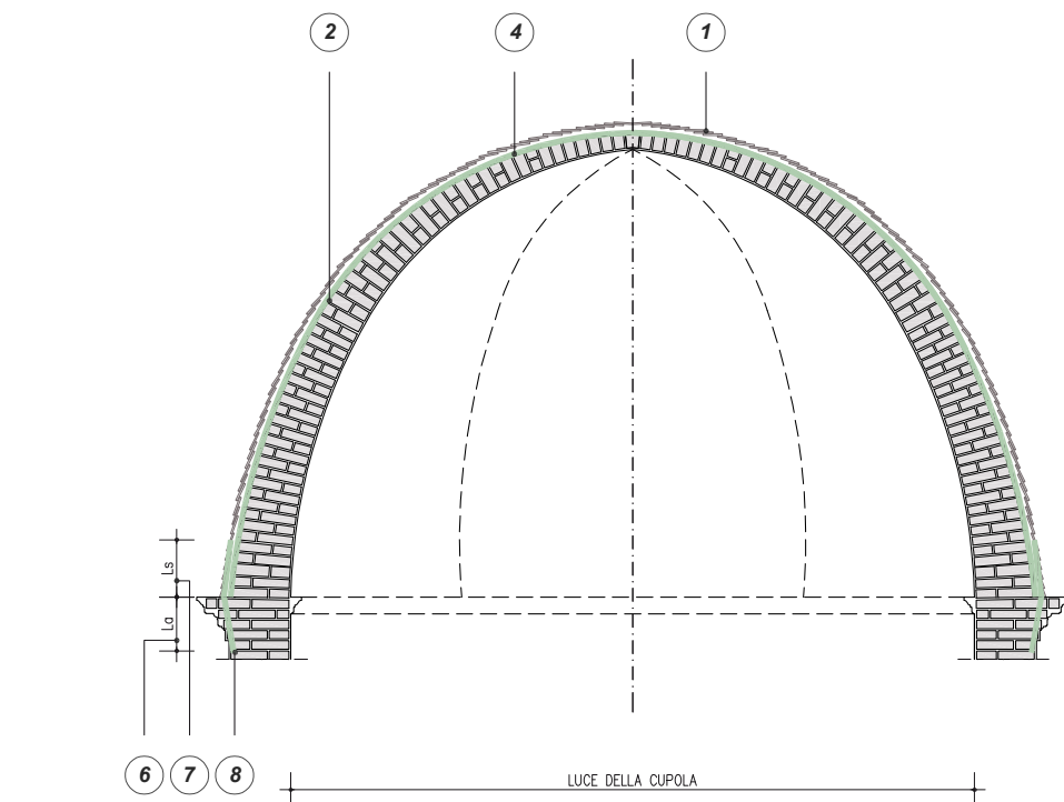
SEZIONE A-A' SISTEMI DI RINFORZO ALL'ESTRADOSSO CON RETE DIFFUSA GEOSTEEL GRID 200/400 O RINFORZO ARV 100
