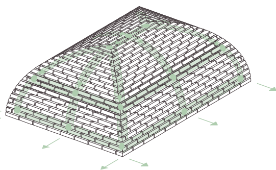
ASSONOMETRIA RINFORZO INTRADOSSALE DELLA VOLTA A PADIGLIONE
