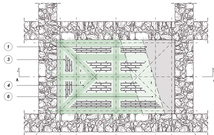
PIANTA SISTEMI DI RINFORZO ALL'ESTRADOSSO CON FASCE DI GEOSTEEL G600/G1200
