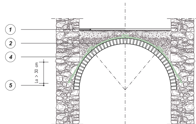
SEZIONE A-A' SISTEMI DI RINFORZO ALL'ESTRADOSSO CON FASCE DI GEOSTEEL G600/G1200
