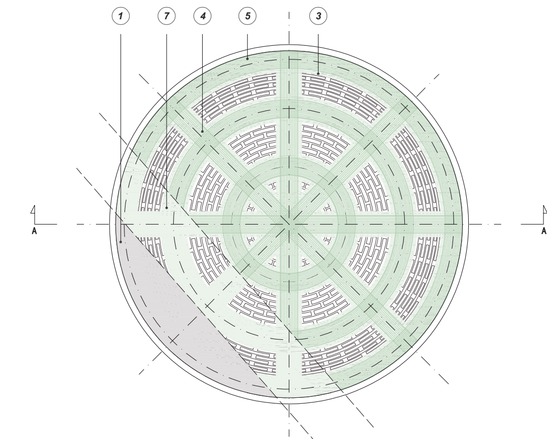
PIANTA SISTEMI DI RINFORZO ALL'ESTRADOSSO CON FASCE DI GEOSTEEL G600/G1200
