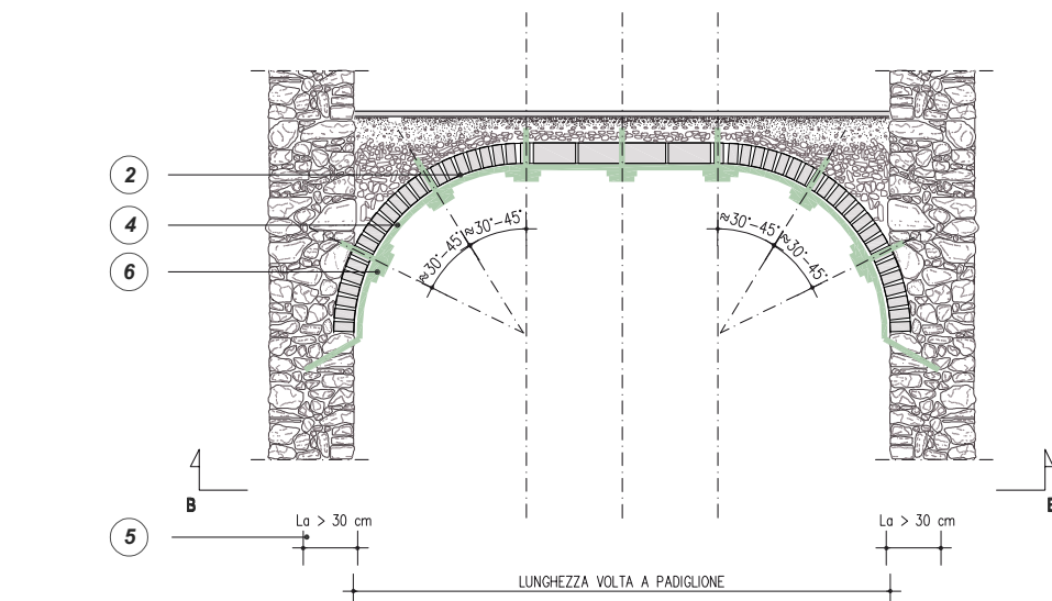
SEZIONE A-A' SISTEMI DI RINFORZO ALL'INTRADOSSO CON FASCE DI GEOSTEEL G600/G1200
