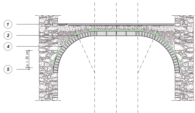
SEZIONE A-A' SISTEMI DI RINFORZO ALL'ESTRADOSSO CON FASCE DI GEOSTEEL G600/G1200
