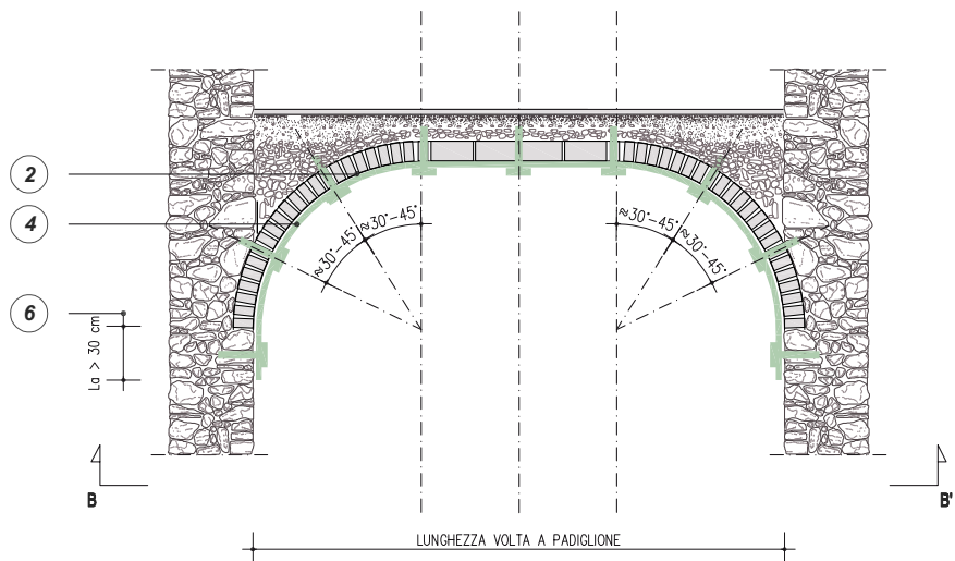
SEZIONE A-A' SISTEMI DI RINFORZO ALL'INTRADOSSO CON RETE DIFFUSA GEOSTEEL GRID 200/400 O RINFORZO ARV 100
