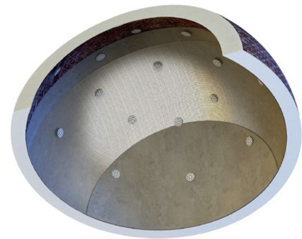
SEZIONE A-A' SISTEMI DI RINFORZO ALL'INTRADOSSO CON RETE DIFFUSA GEOSTEEL GRID 200/400 O RINFORZO ARV 100
