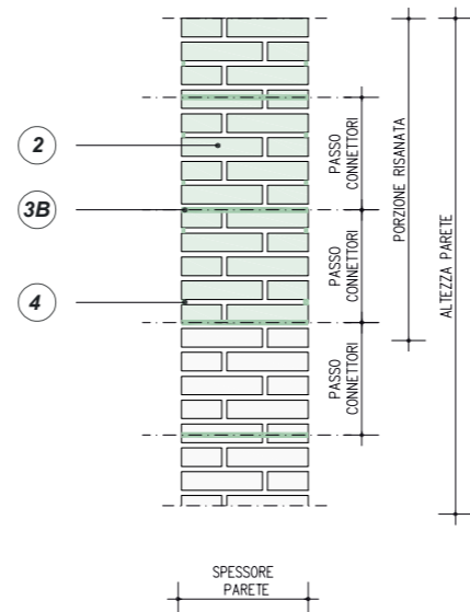
SEZIONE A-A' UNIONE DELL'INTERVENTO DI SCUCI - CUCI CON L'INSERIMENTO DIFFUSO DI CONNESSIONI TRASVERSALI REALIZZATE MEDIANTE BARRE ELICOIDALI STEEL DRYFAST E RISTILATURA ARMATA CON BARRE ELICOIDALI STEEL DRYFAST 6
