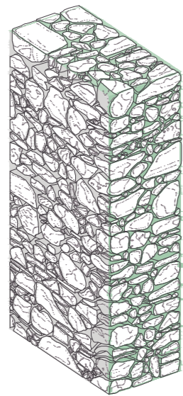
ASSONOMETRIA INIEZIONI DI GEOCALCE FL ANTISMICO
