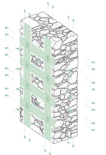
ASSONOMETRIA FASCE IN FIBRA DI ACCIAIO GEOSTEEL G600/G1200
