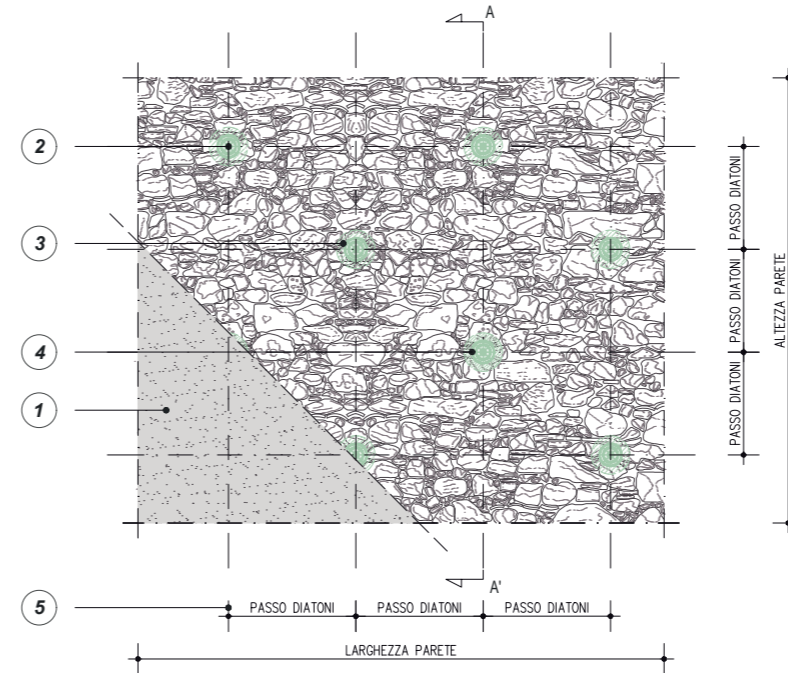
PROSPETTO INSERIMENTO DIFFUSO DI DIATONI ARTIFICIALI A FIOCCO IN FIBRA DI ACCIAIO GALVANIZZATO GEOSTEEL G600/G1200
