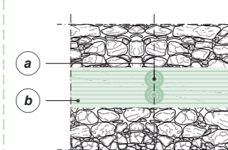
CATENA IN GEOSTEEL G600/G1200 ALLETTATA CON GEOCALCE F ANTISISMICO E INGHISATA ALLA MURATURA CON GEOCALCE FL ANTISISMICO, NELLA ZONA D'ANCORAGGIO
