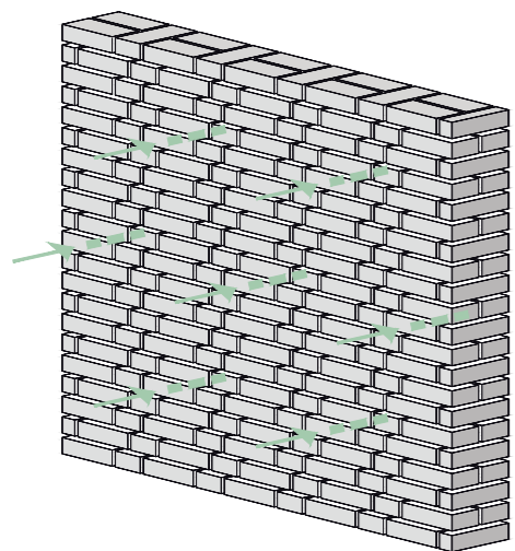
ASSONOMETRIA INSERIMENTO DIFFUSO DI CONNESSIONI TRASVERSALI REALIZZATE MEDIANTE BARRE ELICOIDALI STEEL DRYFAST
