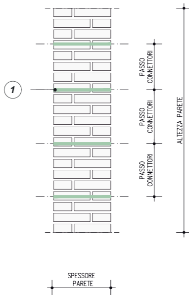
SOLUZIONE CON CONNESSIONI TRASVERSALI PASSANTI
