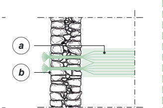
FASCIA DI PIANO IN TESSUTO GEOSTEEL G600/G1200 ALLETTATA CON GEOCALCE F ANTISISMICO
