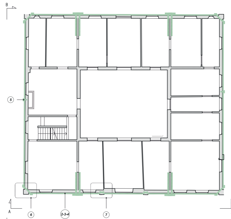
PIANTA RINFORZO DI PORZIONI DI FABBRICATO MEDIANTE FASCE GEOSTEEL G600/G1200
