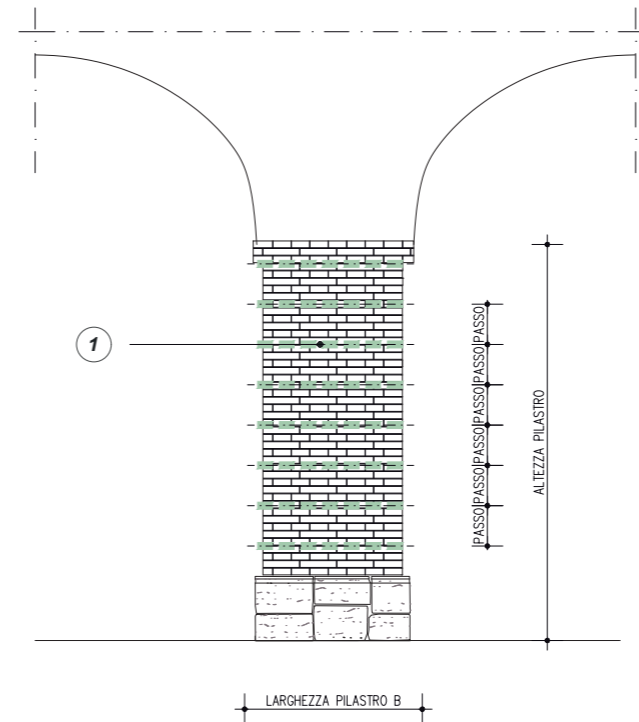
PROSPETTO SEZIONE CIRCOLARE CONFINAMENTO PUNTUALE DEL PILASTRO CON STEEL DRYFAST
