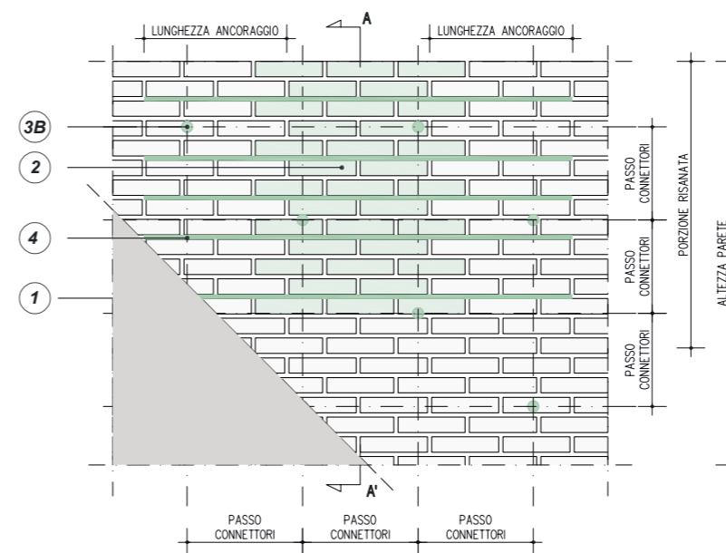
PROSPETTO UNIONE DELL'INTERVENTO DI SCUCI - CUCI CON L'INSERIMENTO DIFFUSO DI CONNESSIONI TRASVERSALI REALIZZATE MEDIANTE BARRE ELICOIDALI STEEL DRYFAST E RISTILATURA ARMATA CON BARRE ELICOIDALI STEEL DRYFAST 6
