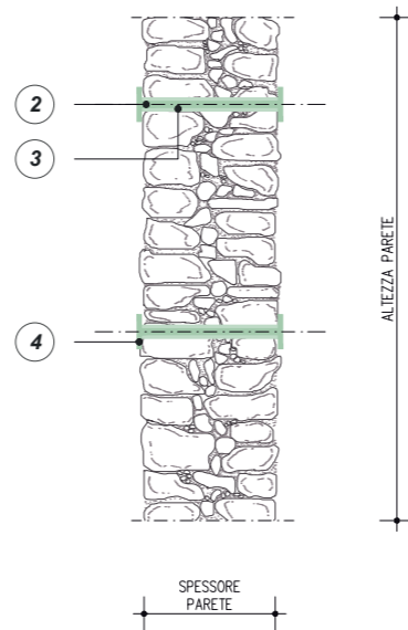
SEZIONE A-A' INSERIMENTO DIFFUSO DI DIATONI ARTIFICIALI A FIOCCO IN FIBRA DI ACCIAIO GALVANIZZATO GEOSTEEL G600/G1200
