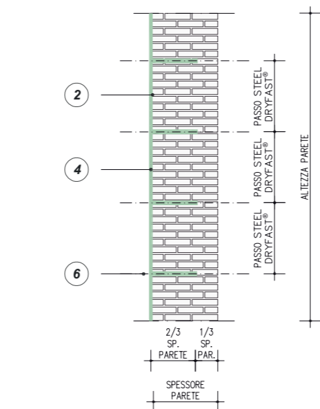
SEZIONE A-A' RINFORZO A FLESSIONE E TAGLIO DEL MASCHIO MURARIO TRAMITE GEOSTEEL GRID 200/400 O RINFORZO ARV 100 SU UN SOLO LATO DEL PARAMENTO
