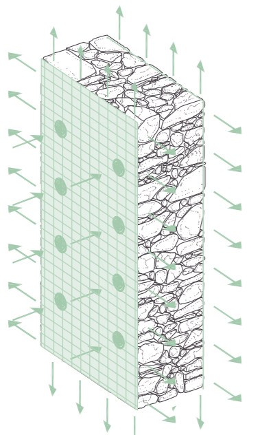
ASSONOMETRIA RETE GEOSTEEL GRID 200/400 O RINFORZO ARV 100
