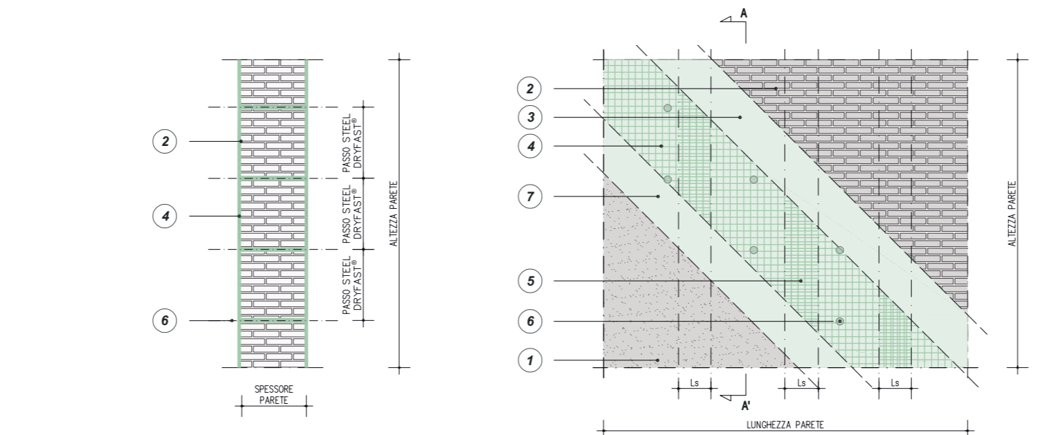
SEZIONE A-A' RINFORZO A FLESSIONE E TAGLIO DEL MASCHIO MURARIO TRAMITE GEOSTEEL GRID 200/400 O RINFORZO ARV 100
