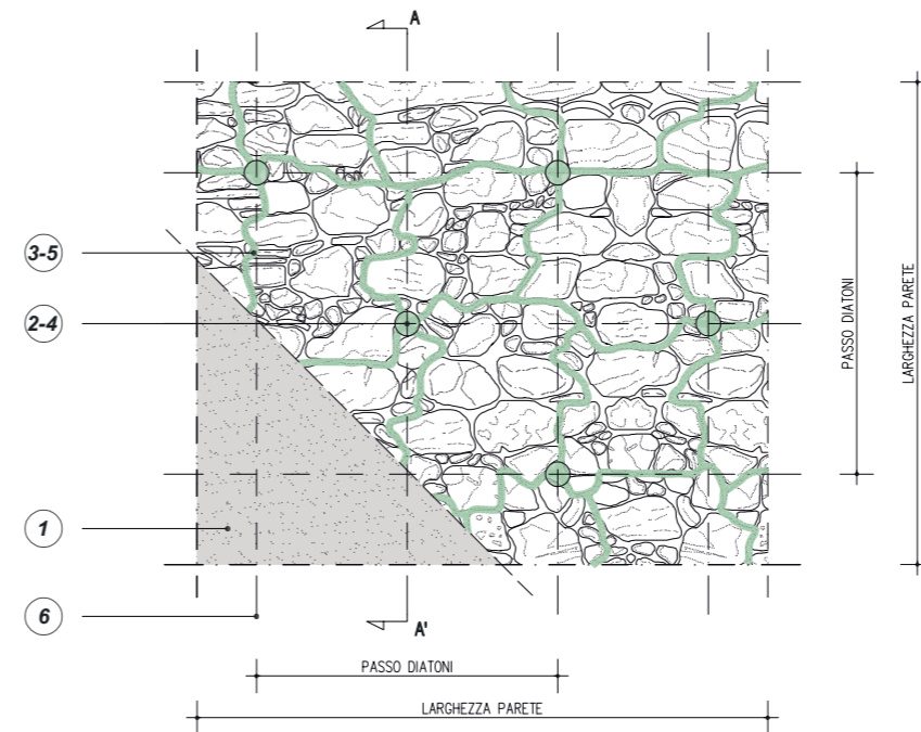
PROSPETTO INSERIMENTO DIFFUSO DI DIATONI ARTIFICIALI A FIOCCO IN FIBRA DI ACCIAIO GALVANIZZATO GEOSTEEL G600/G1200
