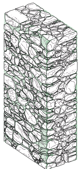
ASSONOMETRIA RISTILATURA PROFONDA DEI GIUNTI
