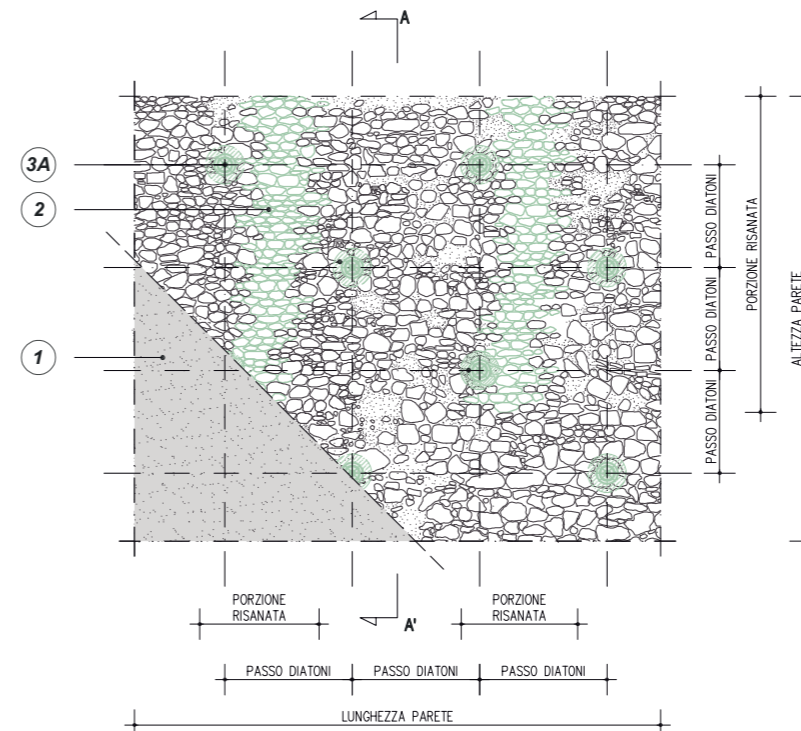
PROSPETTO UNIONE DELL'INTERVENTO DI SCUCI - CUCI CON L'INSERIMENTO DIFFUSO DI DIATONI ARTIFICIALI A FIOCCO IN FIBRA DI ACCIAIO GALVANIZZATO GEOSTEEL G600/G1200
