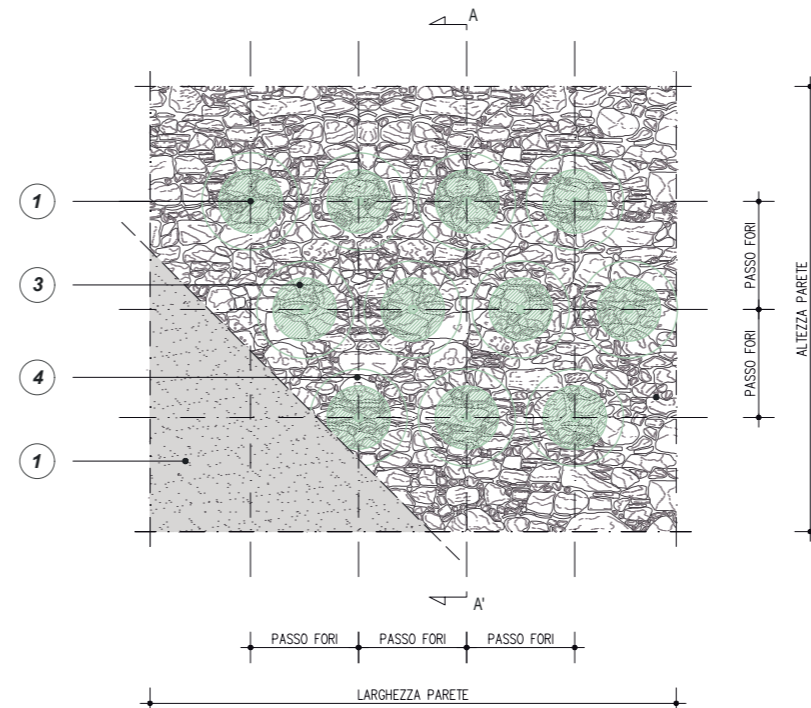
PROSPETTO CONSOLIDAMENTO TRAMITE INIEZIONI DI GEOCALCE FL ANTISMICO
