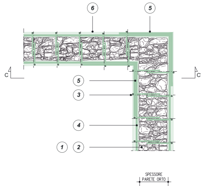
PIANTA RINFORZO PER AZIONI STATICHE DEL MASCHIO MURARIO TRAMITE GLASS NET, BARRE A "L" IN FIBRA DI VETRO GLASS CONNECT L E ANGOLARE GLASS NET A305 SU AMBO I LATO DI PARAMENTI ORTOGONALI TRA LORO
