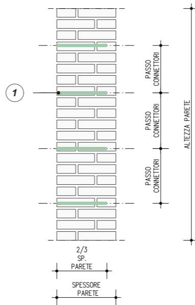
SOLUZIONE CON CONNESSIONI TRASVERSALI NON PASSANTI
