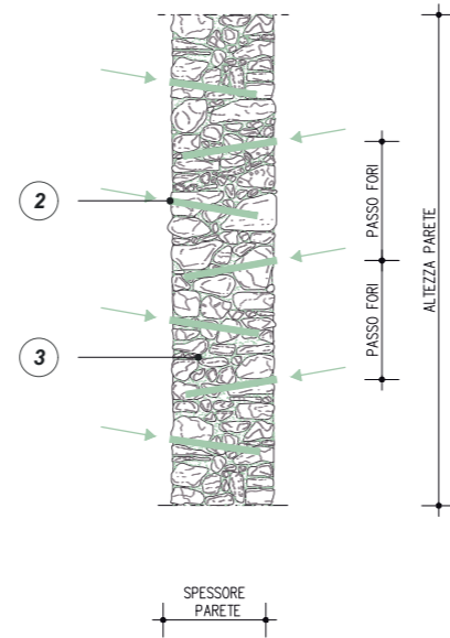
SEZIONE A-A' CONSOLIDAMENTO TRAMITE INIEZIONI DI GEOCALCE FL ANTISMICO
