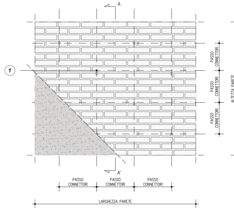
PROSPETTO INSERIMENTO DIFFUSO DI CONNESSIONI TRASVERSALI REALIZZATE MEDIANTE BARRE ELICOIDALI STEEL DRYFAST
