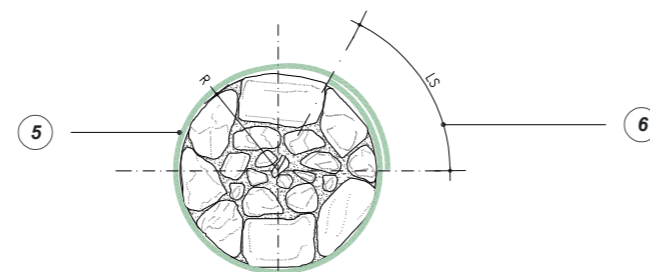
PIANTA SEZIONE CIRCOLARE CONFINAMENTO DEL PILASTRO MEDIANTE FASCIATURA DISCONTINUA CON GEOSTEEL G600/G1200
