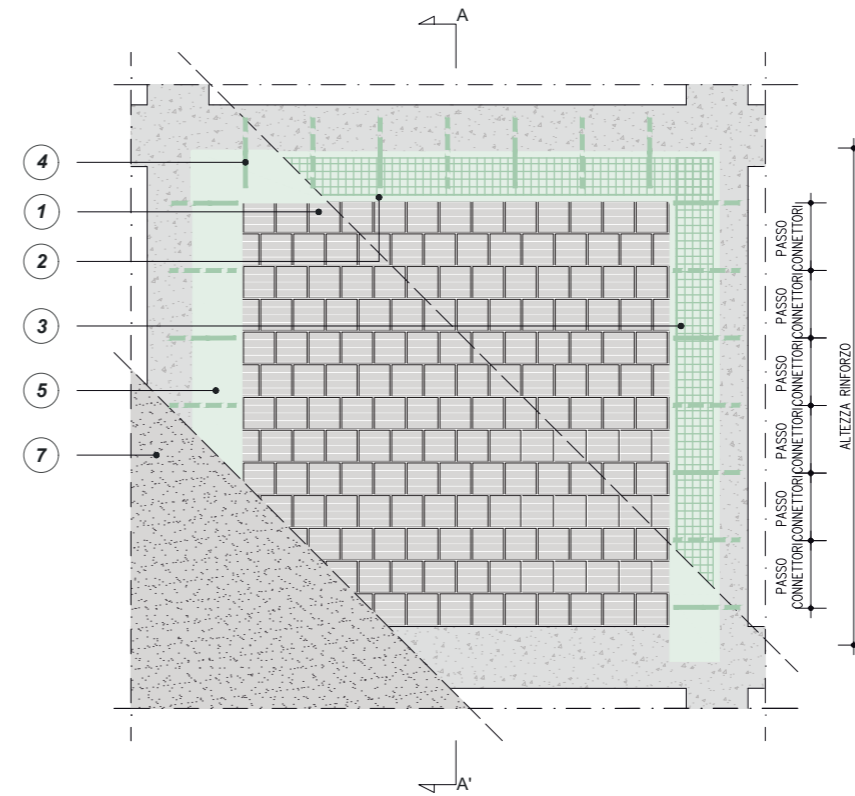
PROSPETTO RINFORZO DELLA TAMPONATURA TRAMITE GEO GRID 120 IN ABBINAMENTO A GEOCALCE F ANTISMICO E BARRE ELICOIDALI IN ACCIAIO INOX
