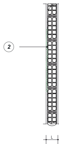
SEZIONE A-A': SITUAZIONE PRE-INTERVENTO RASATURA ARMATA DI MICROLESIONI
