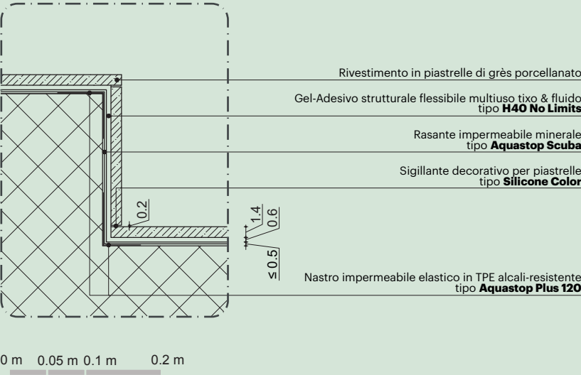
FOCUS RISVOLTO PAVIMENTAZIONE / RIVESTIMENTO
