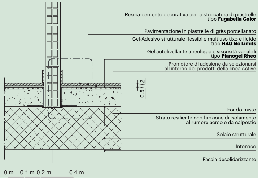
PARTICOLARE COSTRUTTIVO NODO STRATIGRAFIA ORIZZONTALE A PAVIMENTO / DIVISORIO INTERNO A UMIDO
