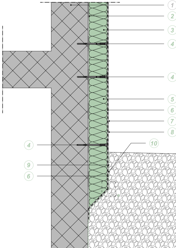
SCALA 1:10
