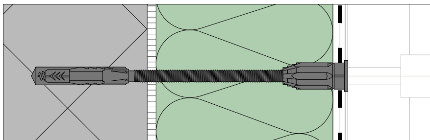
PARTICOLARE A
