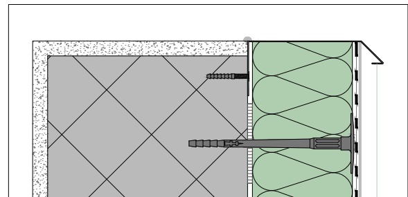
PARTICOLARE A
