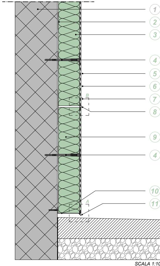
SCALA 1:10
