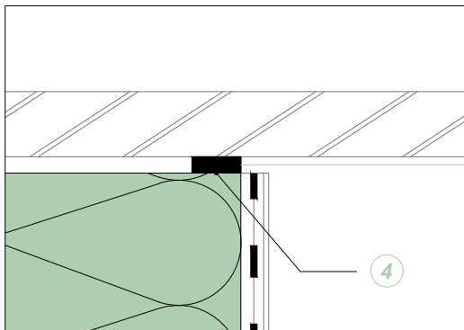
PARTICOLARE A
