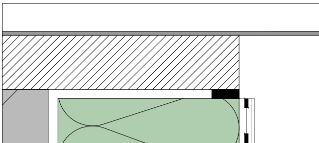
PARTICOLARE A
