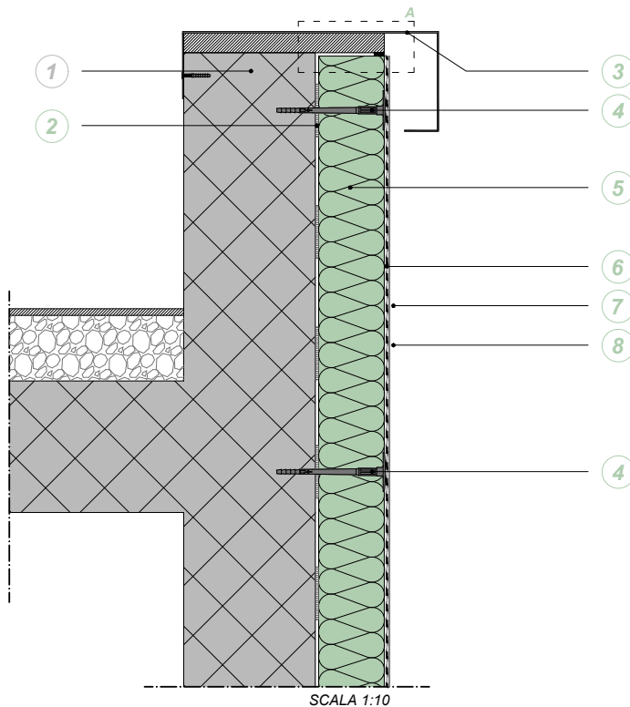
PARTICOLARE A
